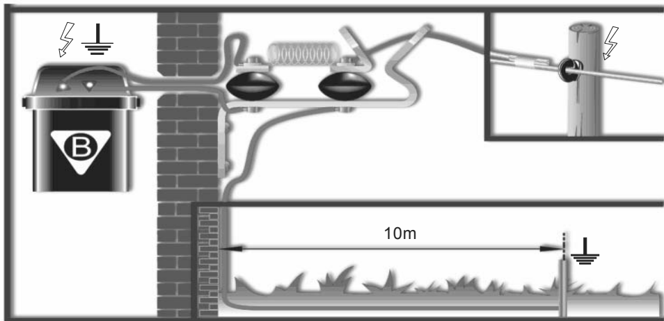
Rys. nr 5 - Sposób podłączenia odgromnika
