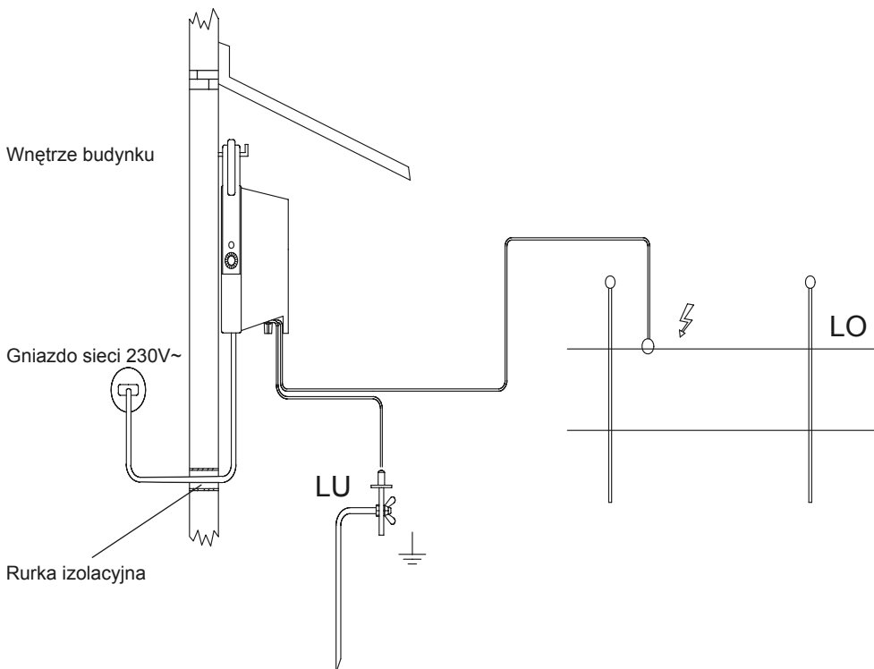
Rys. nr 4 - Sposób instalowania elektryzatora sieciowego EBS-872/M1 zasilanego z sieci 230V~50Hz („LU” – linia uzziemienia, „LO” – linia ogrodzenia)
